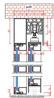
Montaż do sufitu (system Standard – skrzydło + fix)
