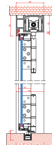
Sama prowadnica dolna „zatopiona” w podłodze.
