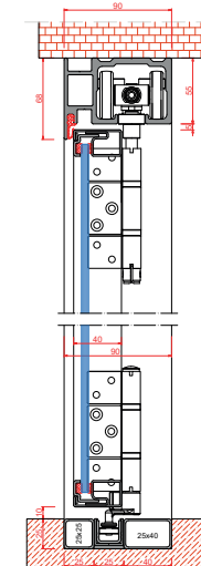
Standardowa rama „zatopiona” w podłodze.
