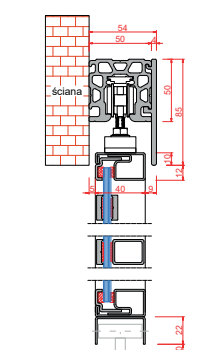
Montaż do ściany/ nadproża (system STANDARD)
