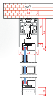
Montaż do sufitu (system STANDARD)
