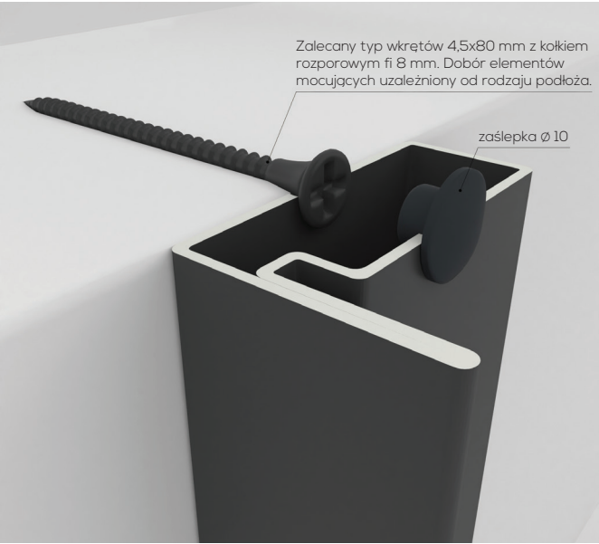
Montaż ościeznicy drzwi rozwiernych
