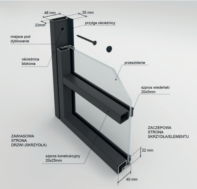
Przekrój ościeznicy oraz skrzydła ze szprosem konstrukcyjnym
