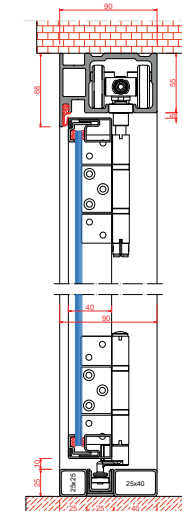
Standardowa rama „leżąca” na podłodze.
