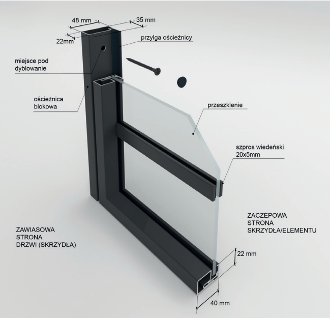
Przekrój ościeznicy oraz skrzydła ze szprosem wiedeńskim
